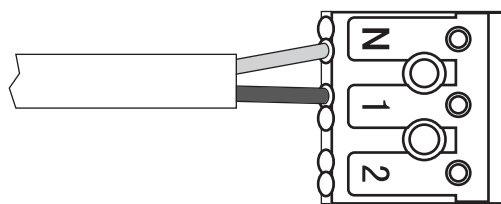
Leuchte - mit Sensor luminaire- with Sensor
